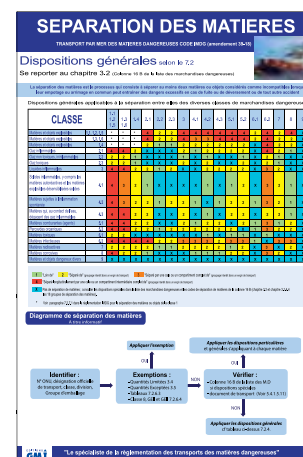
La séparation des marchandises dangereuses selon l'IMDG
