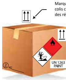
Etiquette 10x10 cm Emballage homologué
